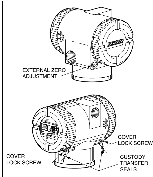
Figure 24. Options -Z1 to -Z3
