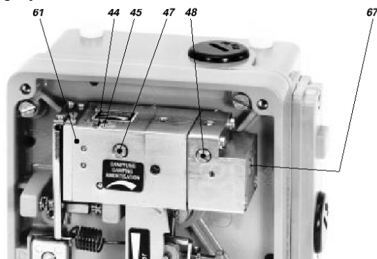
Pozicioner dvostranog dejstva SRI986
