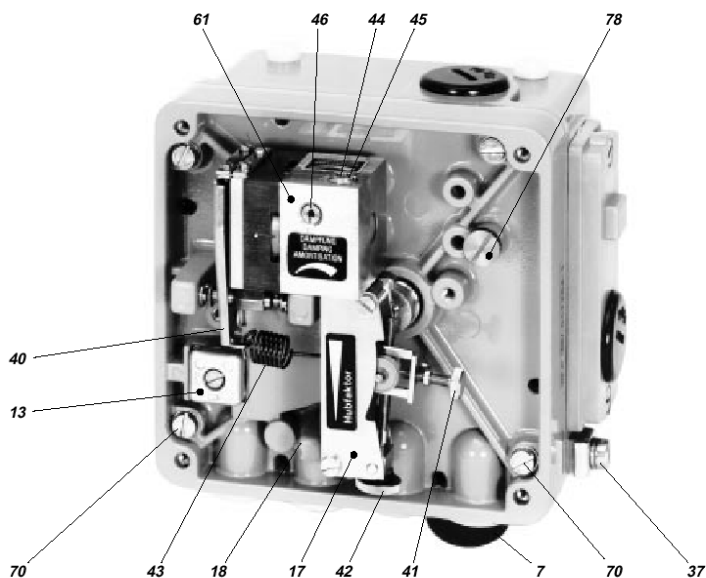
Pozicioner dvostranog dejstva SRI986
