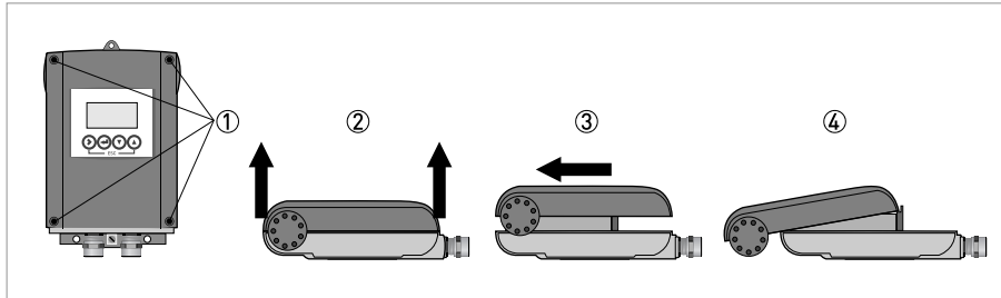
Abbildung 4-7: Öffnen und Schließen des Aluminiumgehäuses
