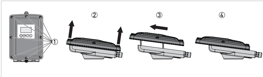
Abbildung 4-8: Öffnen und Schließen des Edelstahlgehäuses
