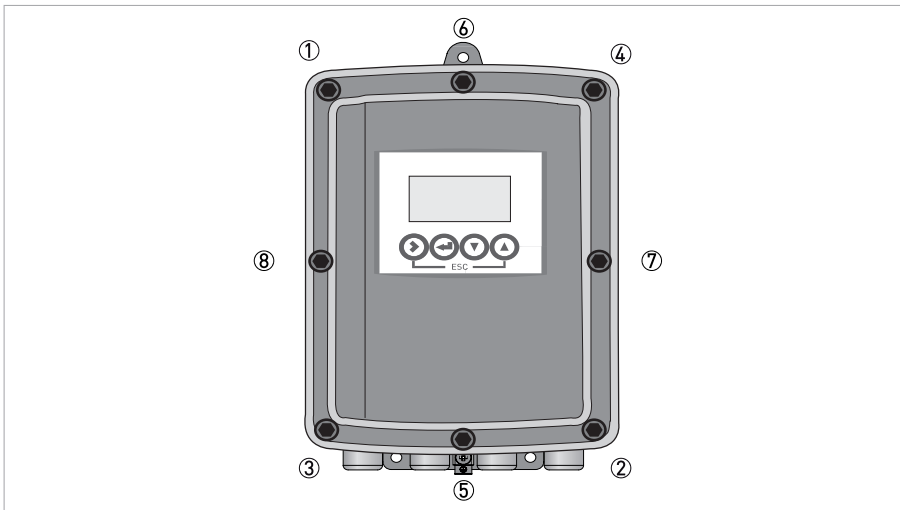
Abbildung 4-9: Ziehen Sie die Schrauben fest.
