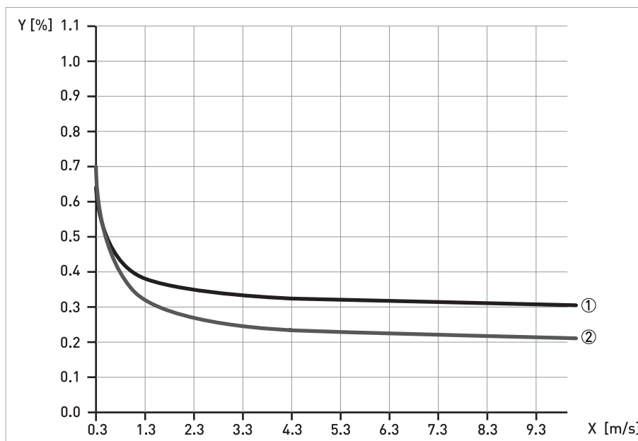
Abbildung 8-8: Messgenauigkeit
