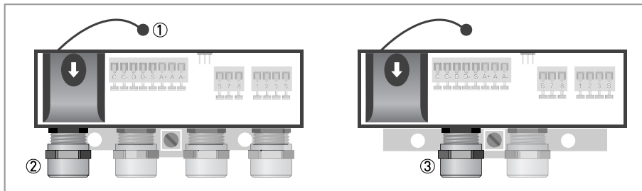
Abbildung 4-13: Anschlussraum Hilfsenergie
