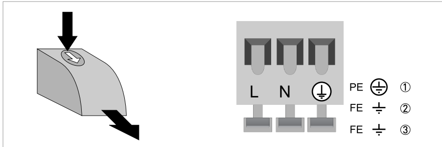
Abbildung 4-14: Anschluss der Hilfsenergie
