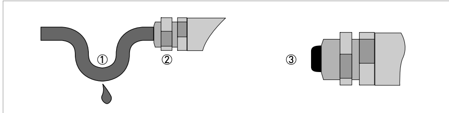
Abbildung 4-17: Gehäuse vor Staub und Wasser schützen
