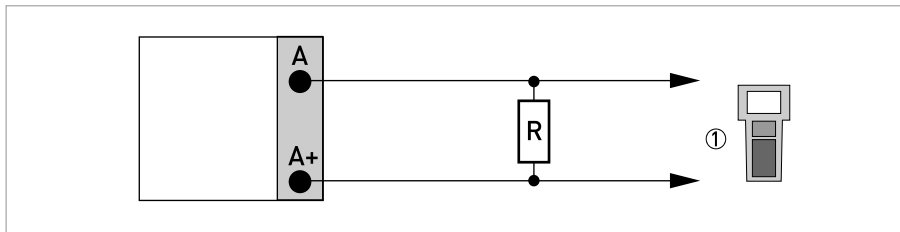
Abbildung 4-23: HART ® -Anschluss aktiv (I a )
