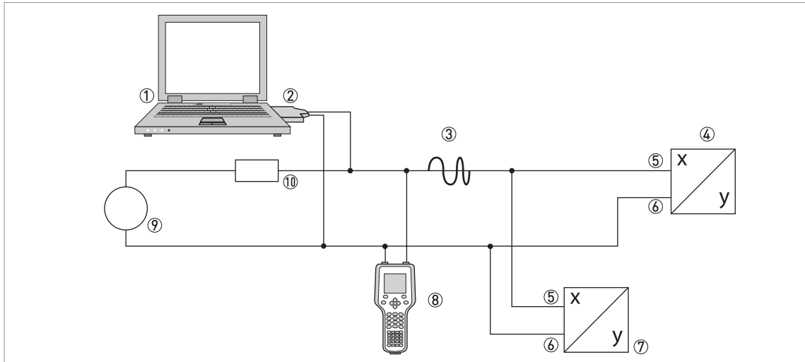
Abbildung 9-2: Multi-Drop-Verbindung (2-Leiteranschluss)
