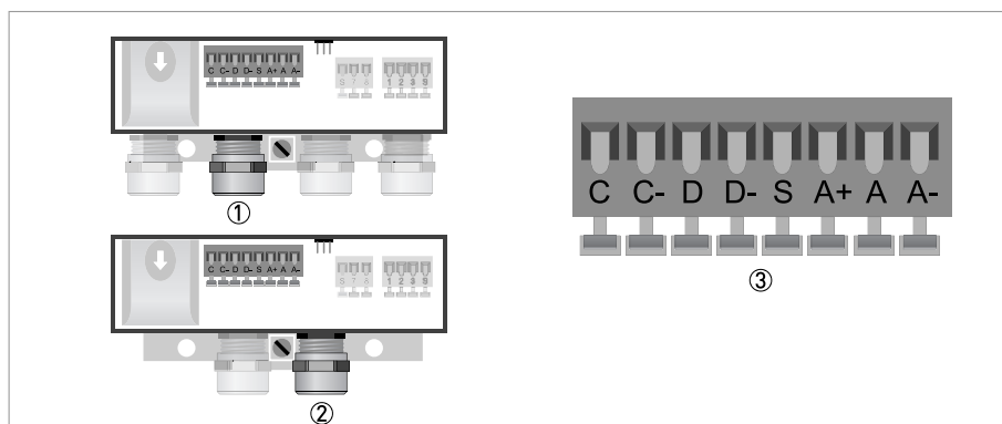
Abbildung 4-16: Anschluss der Ausgänge
